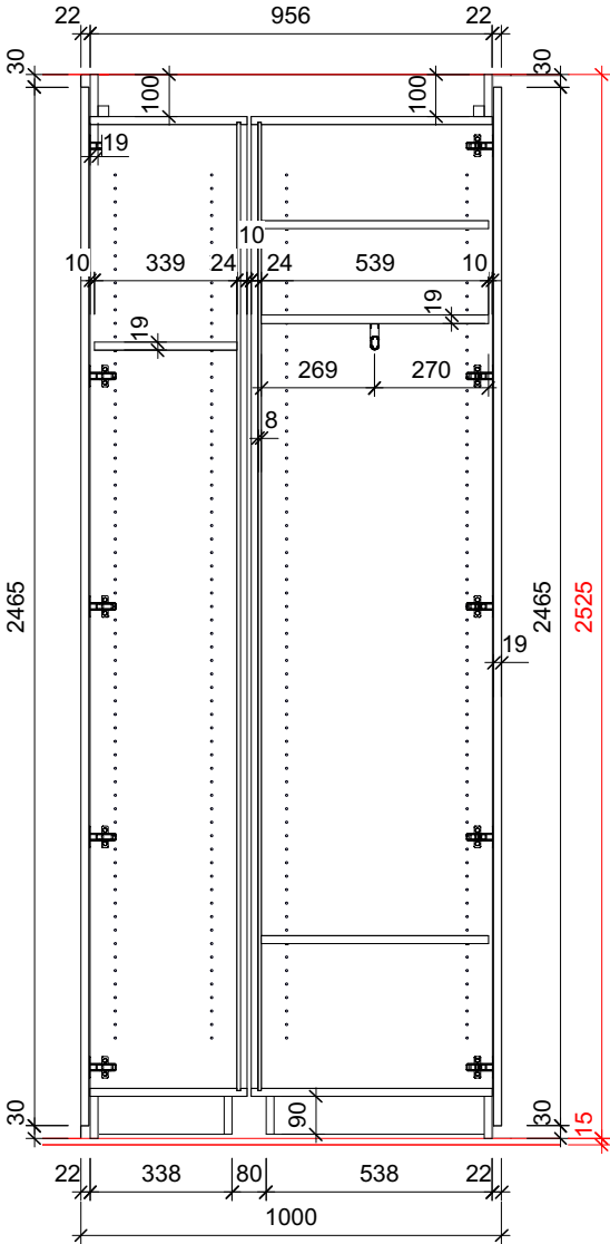
D-D
